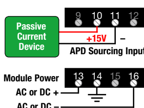
APD 1090 Wiring
