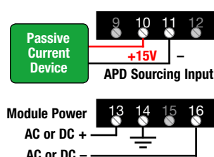
APD 1080 Wiring
